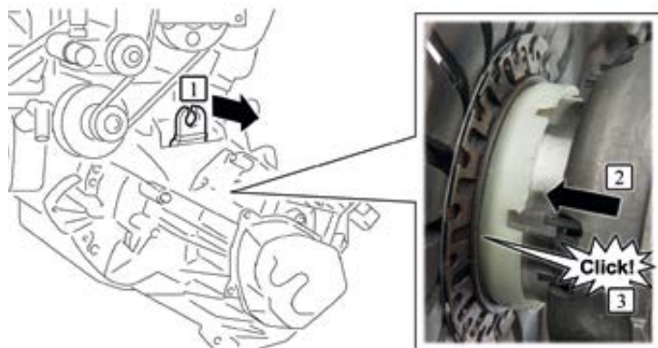
איור 4: עם חזקה חזקה ואגרסיבית של מזלג מיסב הלחץ המיסיב נכנס אל המקום המיועד לו במצמד וניתן לשמוע זאת על ידי רעש ה"קליק" הנלווה.
