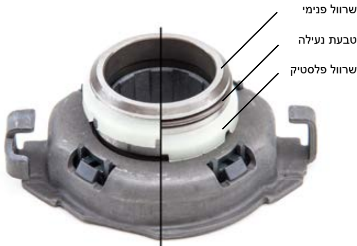
איור 3: טבעת הנעילה במצב מתוח (שמאל) או במצב משוחרר (ימין) על ידי שרוול הפלסטיק.
