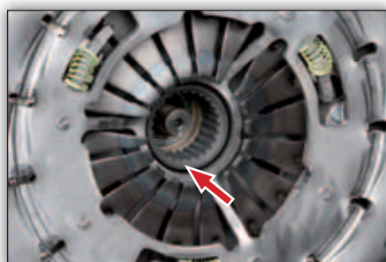
Figur 2: 415 0377 10 med en påmonteret kobling (SAC)
