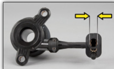
Εικόνα 2: Υδραυλικός σύνδεσμος 13.3 mm για το LuK CSC 510 0097 10
