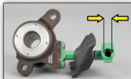
Εικόνα 4: Υδραυλικός σύνδεσμος 12.2 mm για το LuK CSC 510 0137 10
