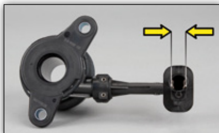
Εικόνα 1: Υδραυλικός σύνδεσμος 12.2 mm για το LuK CSC 510 0090
