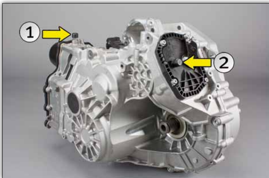
Снимка 1: Скоростна кутия с директна смяна на скорости, с вентилиращи капачки за „мехатроник“ (1) и скоростна кутия (2).
