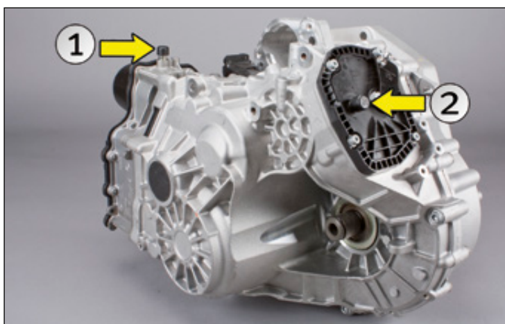
Obrázek 1: Převodovka s přímým řazením s odvzdušňovacími krytkami pro Mechatronik (1) a převodovku (2)
