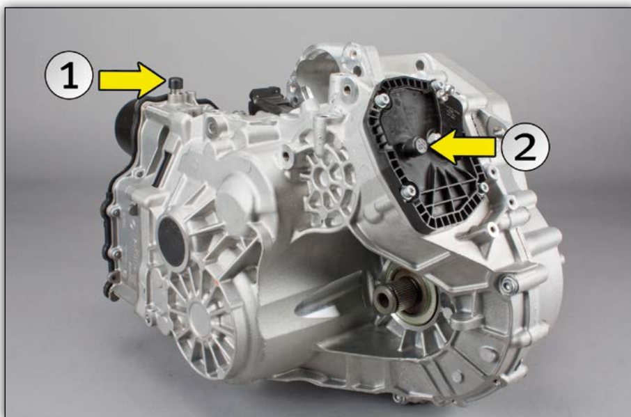
1. ábra: Közvetlen kapcsolású sebességváltó szellőzőkupakkal a mechatronika (1) és a sebességváltó (2) számára
