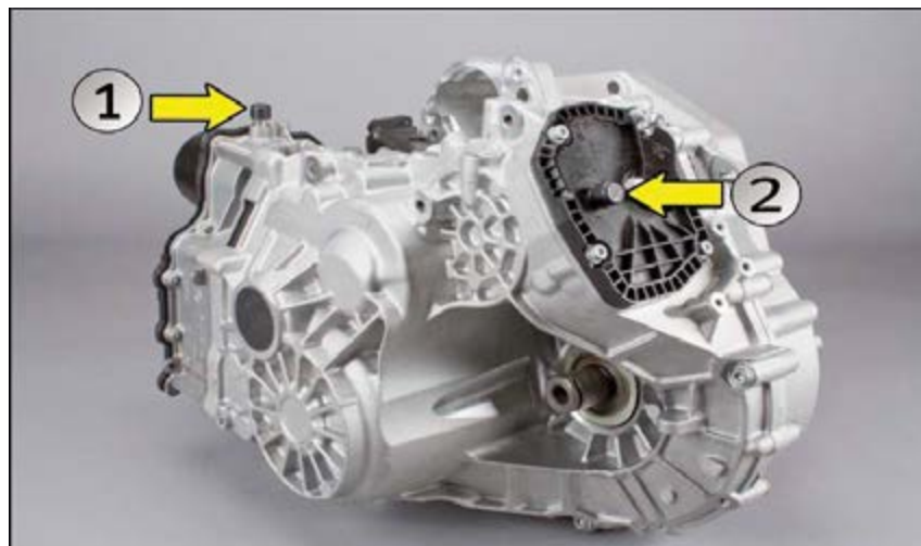
Рис. 1: Преселективная коробка передач - вентиляционные колпачки на блоке мехатроники (1) и КПП (2)
