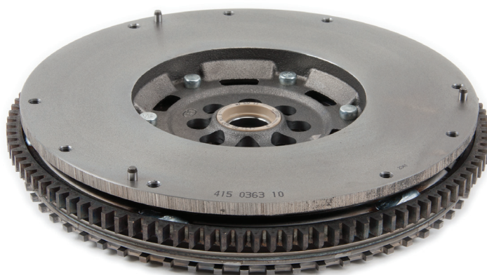
Fig. 1: Tweedelig vliegwiel van LuK 415 0363 11
