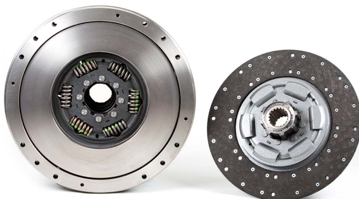
Bild 3: Exempel på dubbellamellkoppling med olika navkonstruktioner
