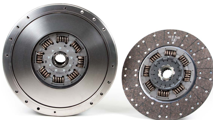
Bild 2: Dubbellamellkoppling från LuK med samma navprofiler
