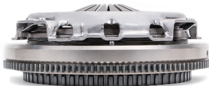
Photo 1 : Lors du montage, les goupilles de centrage n'entrent pas dans les alésages
