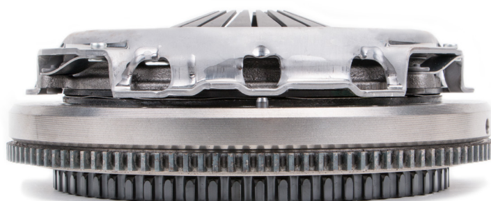
Fig. 1: De centreerstiften komen bij de montage niet in de openingen te zitten
