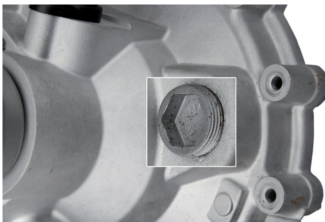
Bild 1: Ausführung der Öleinfüllschraube mit Innensechskant
