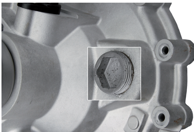
Fig. 1: Uitvoering van de olievlugplug met binnenzeskant
