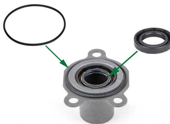
Geleidingsbus met voormonteerde O-ring en keerring
