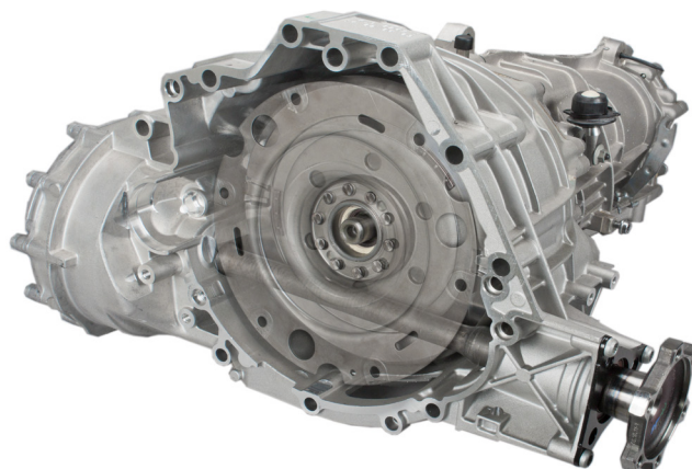
Obrázek 1: Spojovací hřídel přední nápravy probíhá mezi přenosovým plechem a dvoumotovým setrvačником
