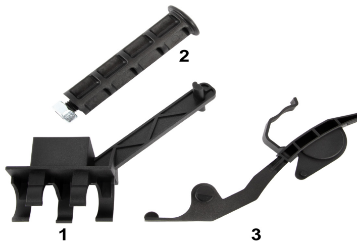
Obrázek 2: Sada montážních přípravků s objednacím číslem 400 0537 10
