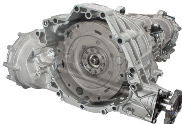
Bild 1: Framaxelns flänsaxel löper mellan drivplattan och dubbelmassasvänghjulet
