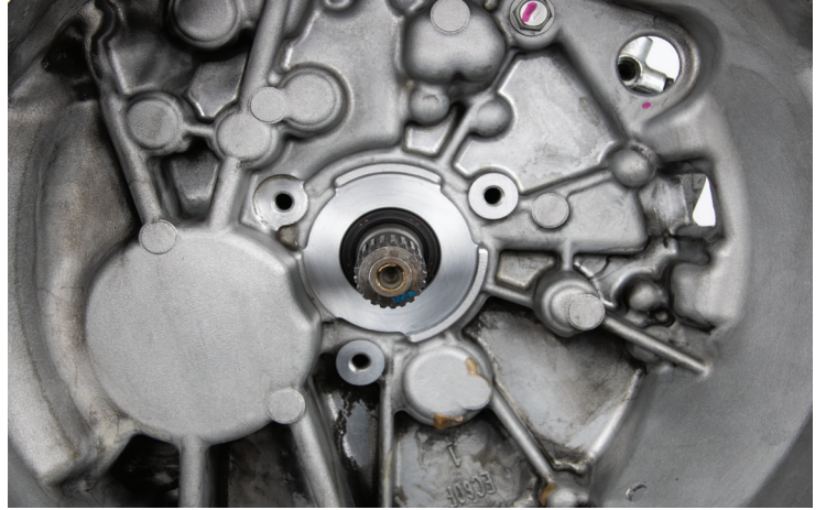
Resim 1: Şanzıman gövdesindeki hidrolik debriyaj rulmanı temas alanı
