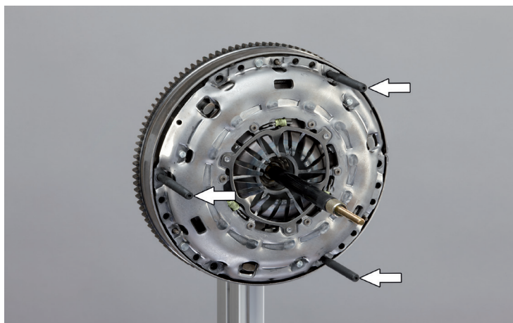
Fig. 2: Espárrago para el alojamiento del soporte del husillo
