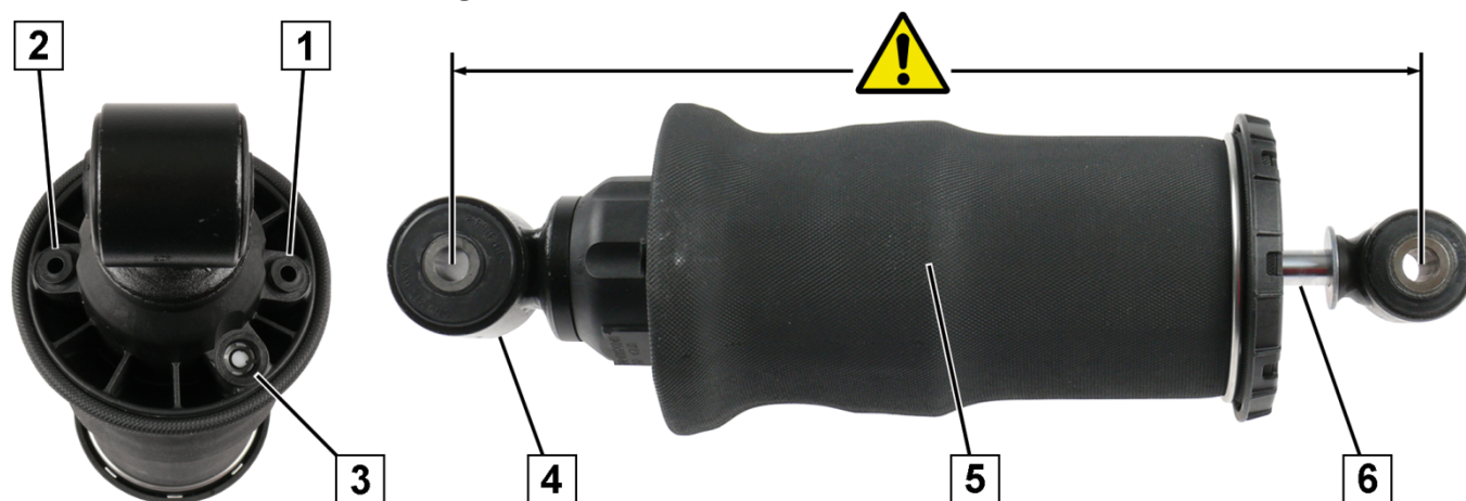
Fig.1: CALM (Cabin Air Leveling Module) mit 2 Anschlüssen / with 2 connetions / avec 2 raccords / con dos conexiones
