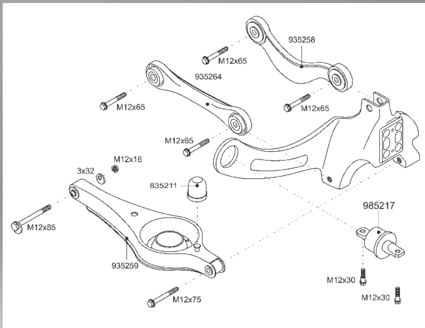
Imagen 1: sección 935259S (fig.: lado izquierdo del vehículo)
