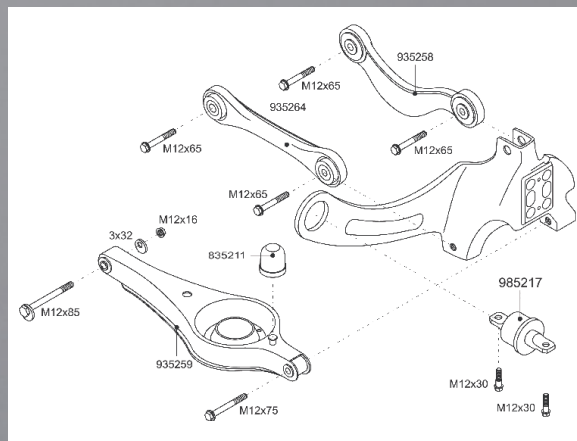
Imagen 1: sección 935259S (figura: lado izquierdo del vehículo), para una vista más grande, véase la página 2
