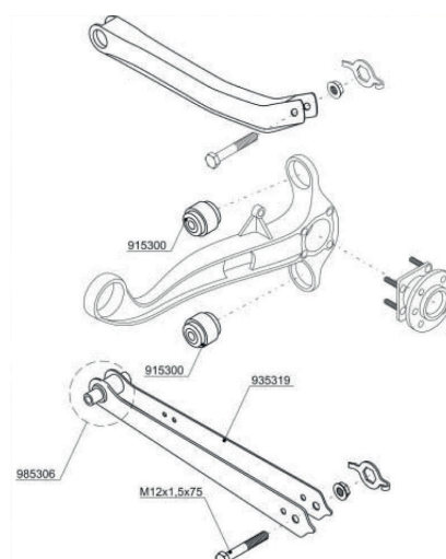
Figure 1: Bielle de train arrière pour Opel Vectra
