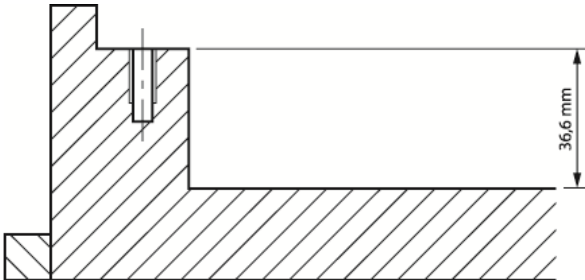
Abb. 1: Schwungrad / Flywheel / Volant Moteur/ Volante del motor
