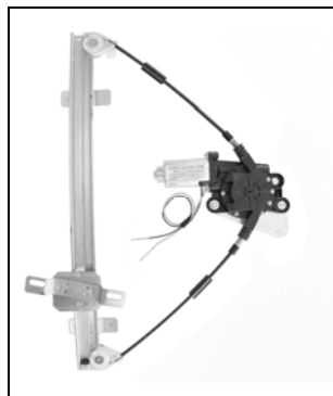
Nuestro elevallunas – notre lève-vitre – our window regulator – nosso levantador de vidro
