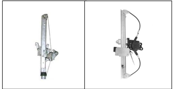
Elevallas original – lève-vitre original – oem window regulator – levandator de vidro original Nuestro elevallas – notre lève-vitre – our window regulator – nosso levantador de vidro
