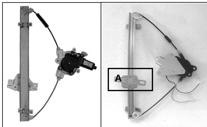
Elevalunas original – lève-vitre original Nuestro elevavinas – notre lève-vitre – oem window regulator – levandator – our window regulator – nosso de vidro original levantador de vidro
