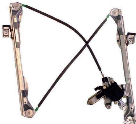
Elevallunas original / OEM window regulator / Lève-vitre original / Elevador de vidro original
