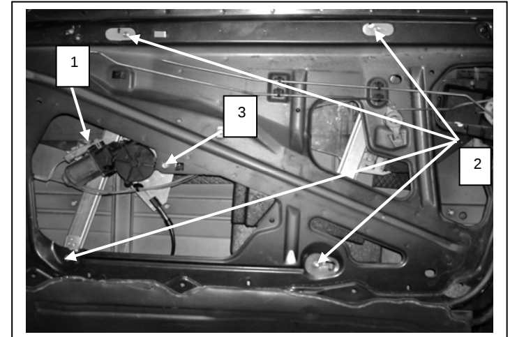
Puerta lado derecho, Portière avant droite, Right front door, Porta frente dirota
