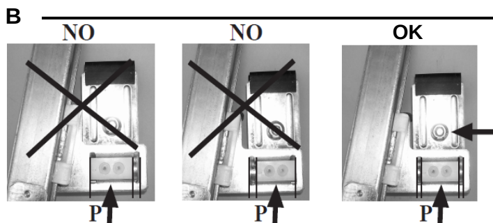
Puerta lado izquierdo, Portière avant gauche, Left front door, Porta frente esquerda
