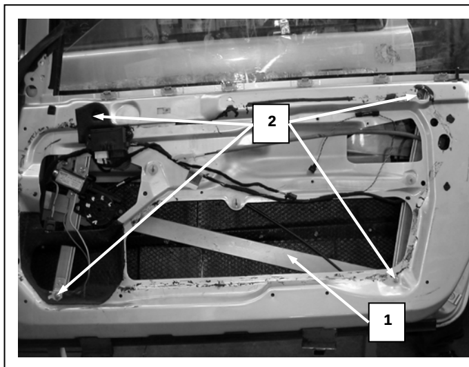
Puerta lado derecho, Portière avant droite, Right front door, Porta frente direita
