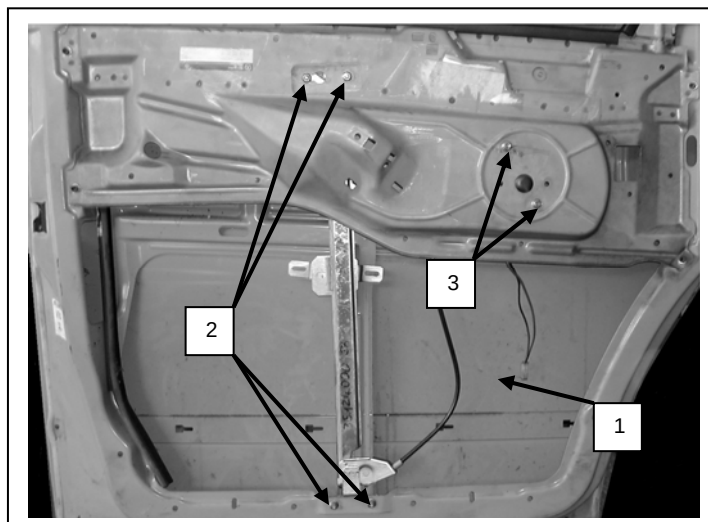
Puerta lado derecho, Portière avant droite, Right front door, Porta frente diáeta
