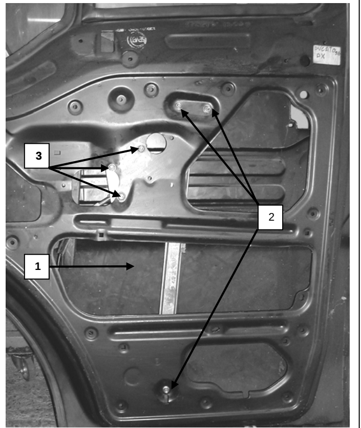
Puerta lado derecho, Portière arrière droite, Right rear door, Porta traseira direita
