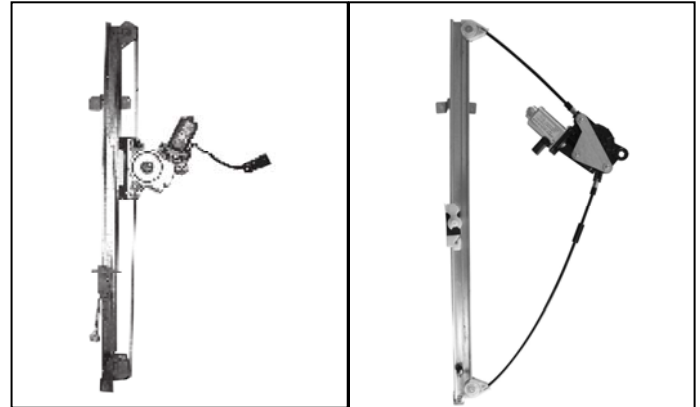
Elevalunas original – lève-vitre original Nuestro elevallunas – notre lève-vitre – oem window regulator – – our window regulator – nosso – levandator de vidro original levandador de vidro μας
