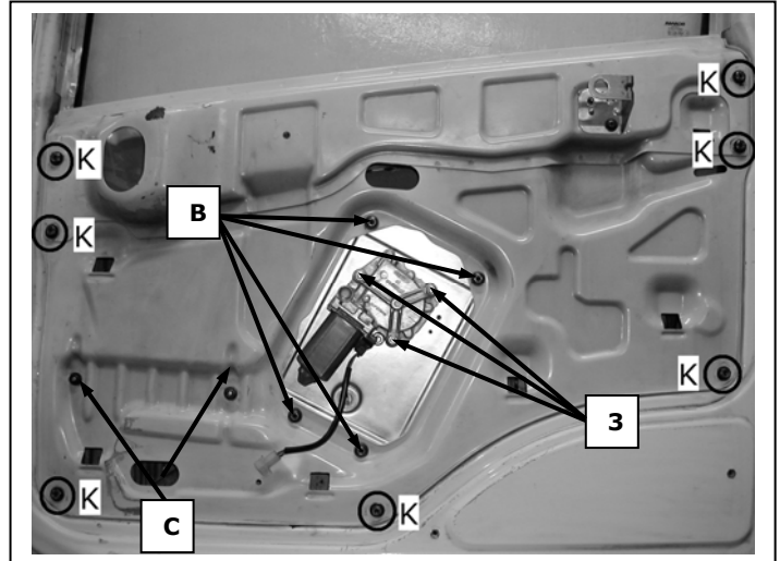
Puerta lado derecho, Portière avant droite, Right front door Porta frente dirieta, Sag on kapi, πόρτα εμπρός δεξιά
