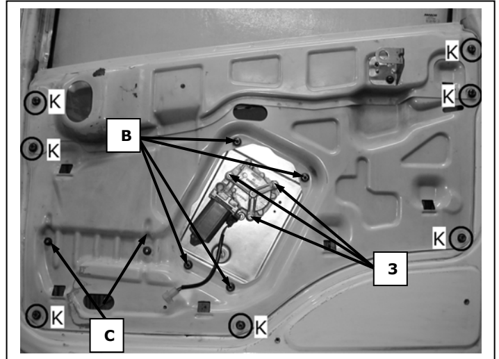
Puerta lado derecho, Portière avant droite, Right front door Porta frente dirieta, Sag on kapi, πόρτα εμπρόσθια δεξιά
