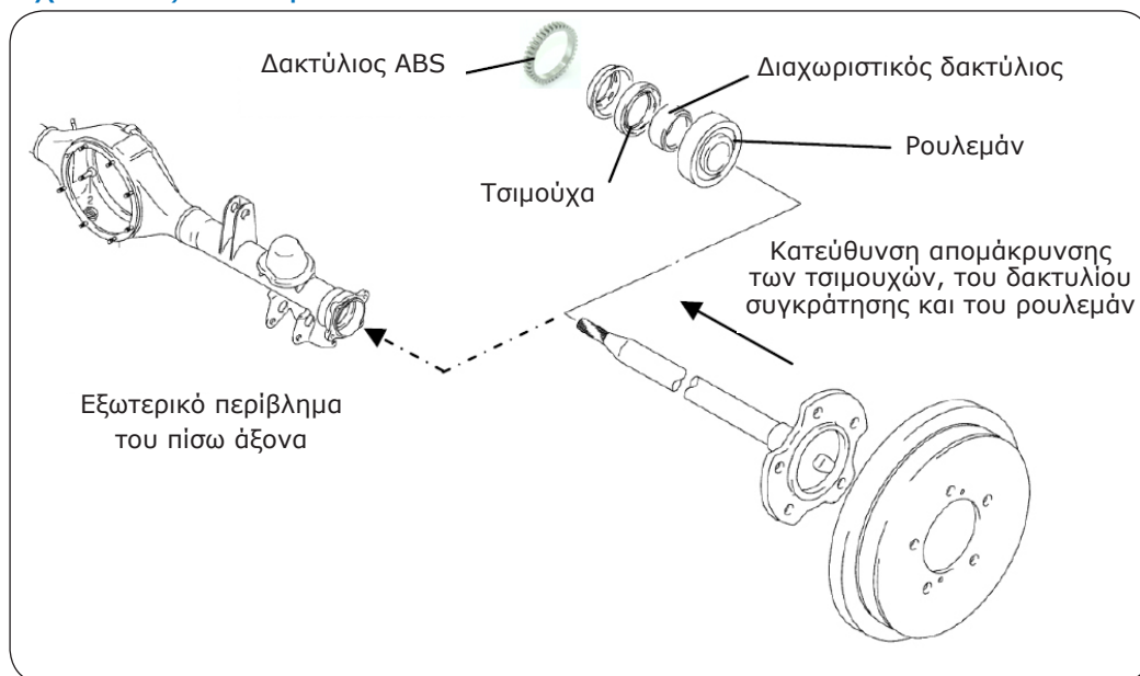
Διαχωριστικός δακτύλιος
