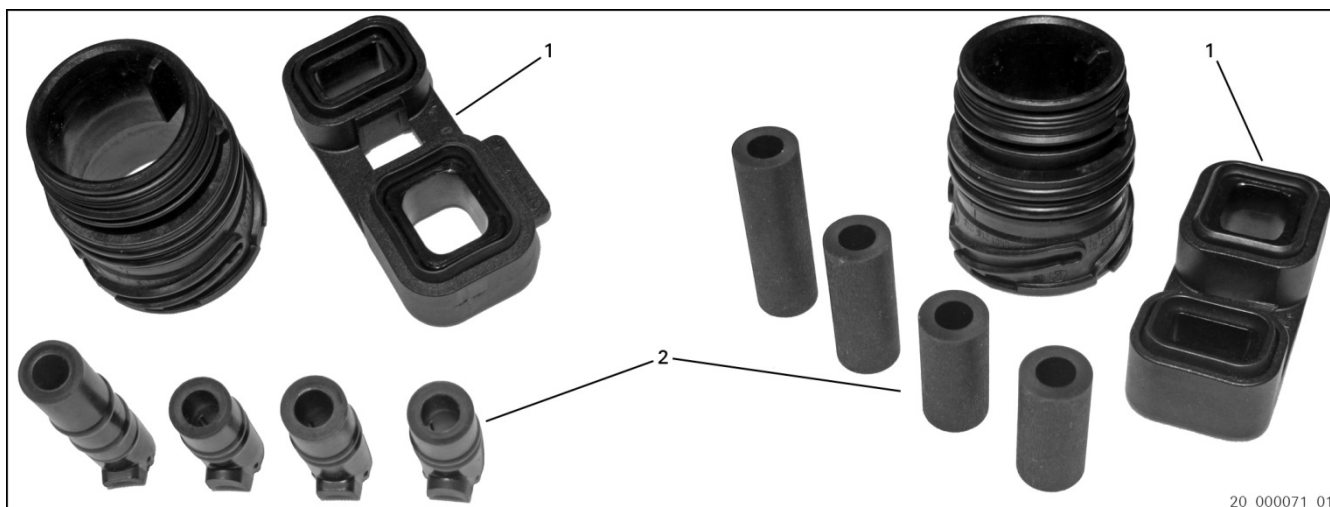
Fig. 1: Jogos de vedações (exemplos)
