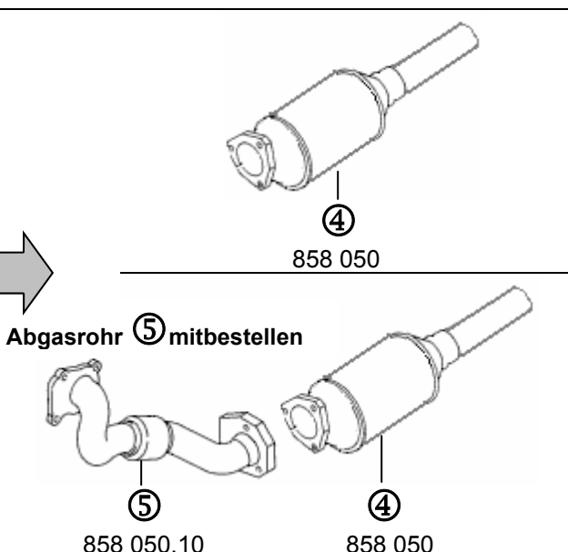
Abb.2: NACHRÜSTUNG mit Partikel-Kat
