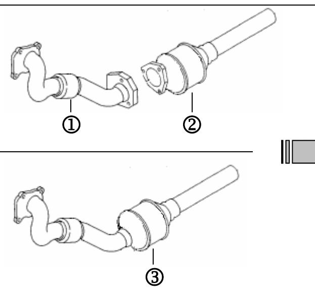
Abb.1: SERIE - Abgasrohr + Serienkatalysator
