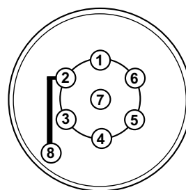
Connecteur des câbles le jack à 7 poles
