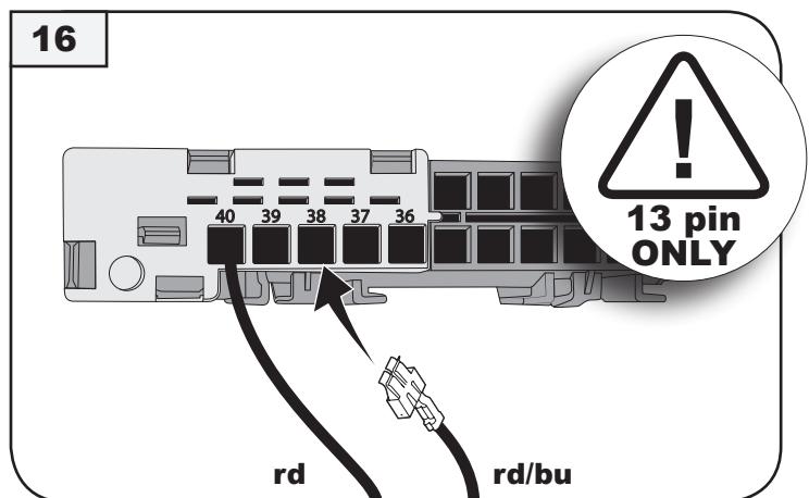
Sicherungskasten fusebox
