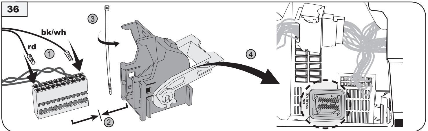
rd → PIN 31 E-Satz Stecker, bk/wh → PIN 39 E-Satz Stecker rd → PIN 31 e-kit socket, bk/wh → PIN 39 e-kit socket
