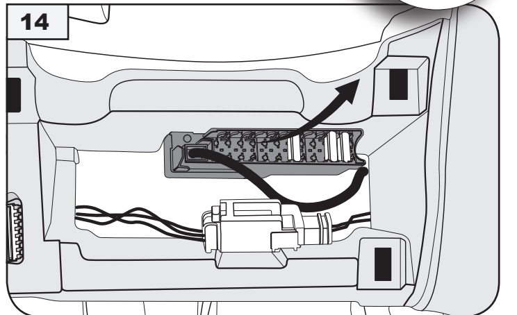
Sicherungskasten fusebox
