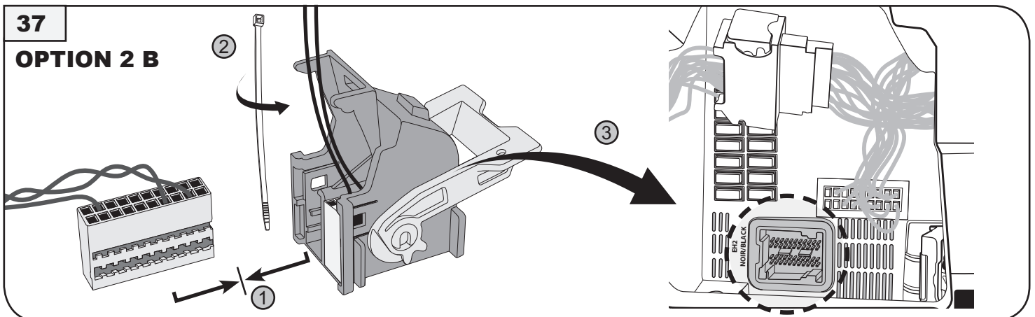
E-Satz Stecker → Fahrzeug Stecker e-kit socket → car socket
