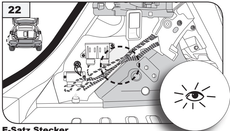
E-Satz Stecker e-kit socket
