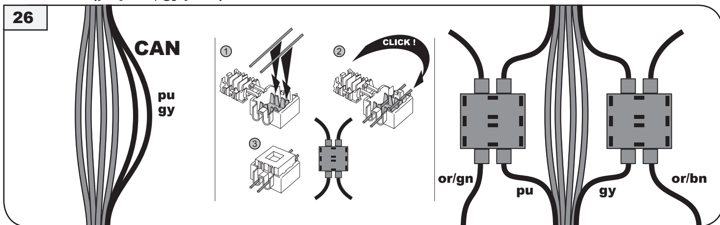
E-Satz Stecker (pu pin 1, gy pin 3) e-kit socket (pu pin 1, gy pin 3)
