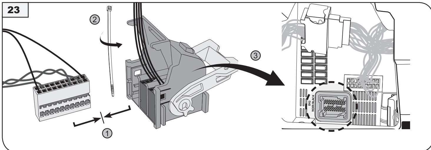
Fahrzeug Stecker car socket
