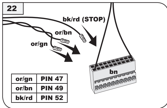
E-Satz → Fahrzeug Stecker e-kit → car socket
