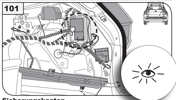
Sicherungskasten fusebox
