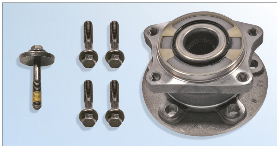
1. ábra: FAG-Kit 713 6186 30
