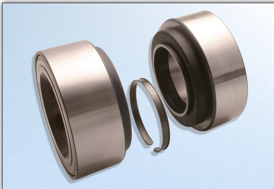
Obrázek 1: Výměnné kompaktní ložisko (RIU)
