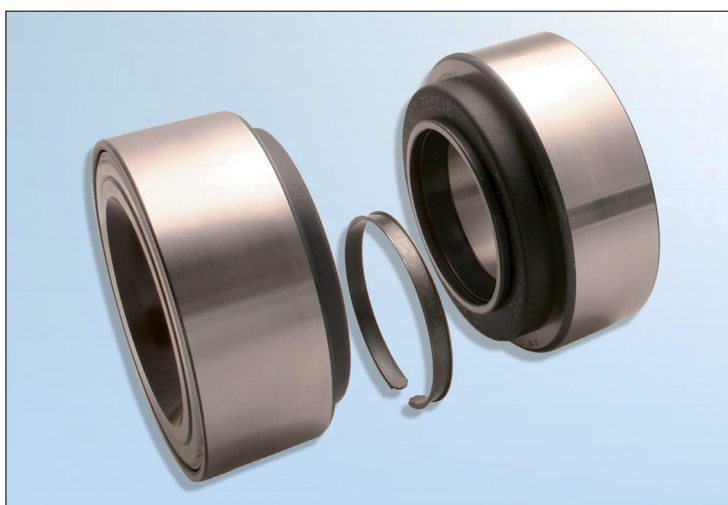
Kuva 1: Vaihdettava laakeri (RIU)
