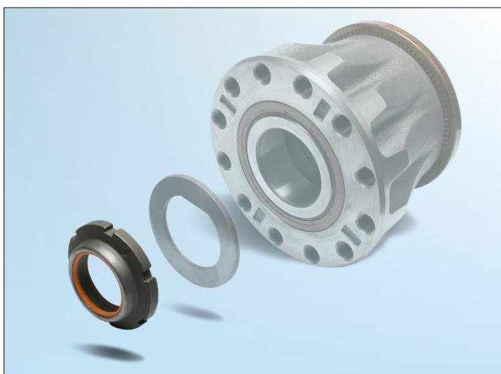
Kuva 1: Akselitapin mutteri 434 0431 10 on saatavana FAG-varusteena.
