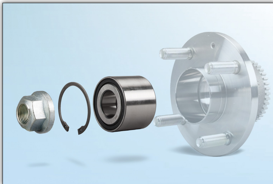
Fig. 1: Kit-ul cu rulmenți de roată FAG 713 6448 00 ca soluție de reparații – butucul nu trebuie înlocuit
