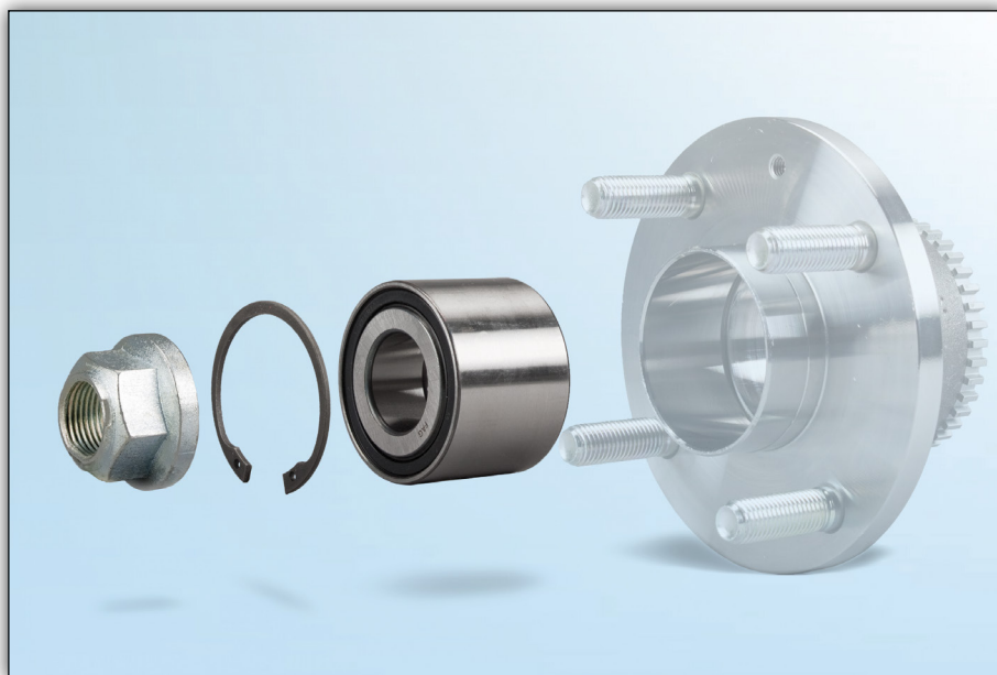
Снимка 1: Комплектът колесен лагер 713 6448 00 на FAG като ремонтно решение — главината на колелото не трябва да се сменя
