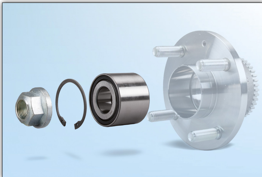
Obrázek 1: FAG sada ložiska kola 713 6448 00 jako řešení pro opravy – náboj kola není nutné vyměňovat.
