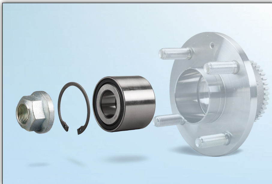
Εικόνα 1: Το σετ ρουλεμάν τροχού FAG 713 6448 00 σαν λύση επισκευής - το άκρο του τροχού δεν πρέπει να αντικατασταθεί
