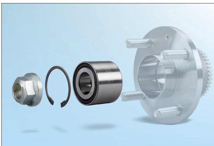
Kuva 1: FAG pyörän laakerisarja 713 6448 00 korjausratkaisuksi – pyörän napaa ei tarvitse vaihtaa.
